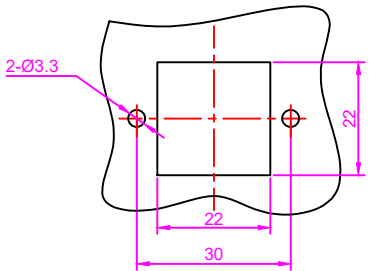
面板开孔图 Panel cut
